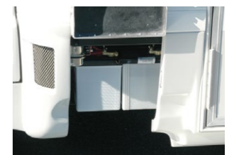
エントランス横のメイン&サブバッテリー
